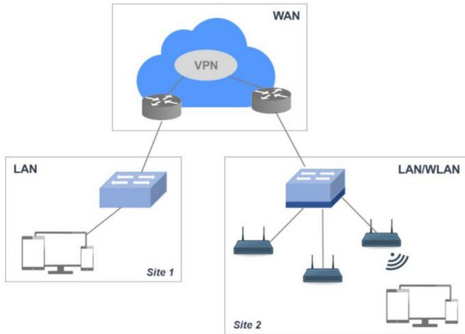
Fig1.- LAN/WAN
